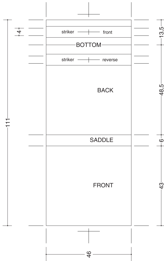
BOOKMATCH DIMENSION CHART · SCALE 1/1 · UNIT m/m
