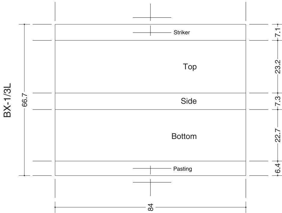
MATCHBOX DIMENSION CHART · SCALE 1/1 · UNIT m/m
