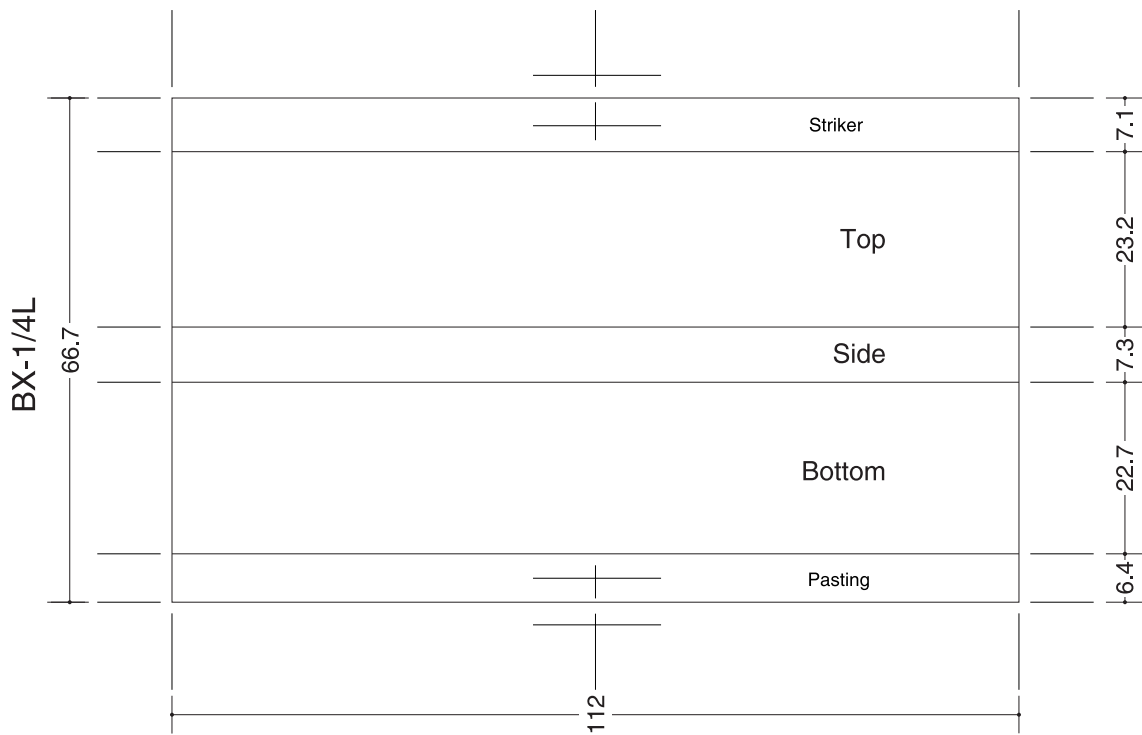
MATCHBOX DIMENSION CHART · SCALE \frac{1}{4} · UNIT m/m
