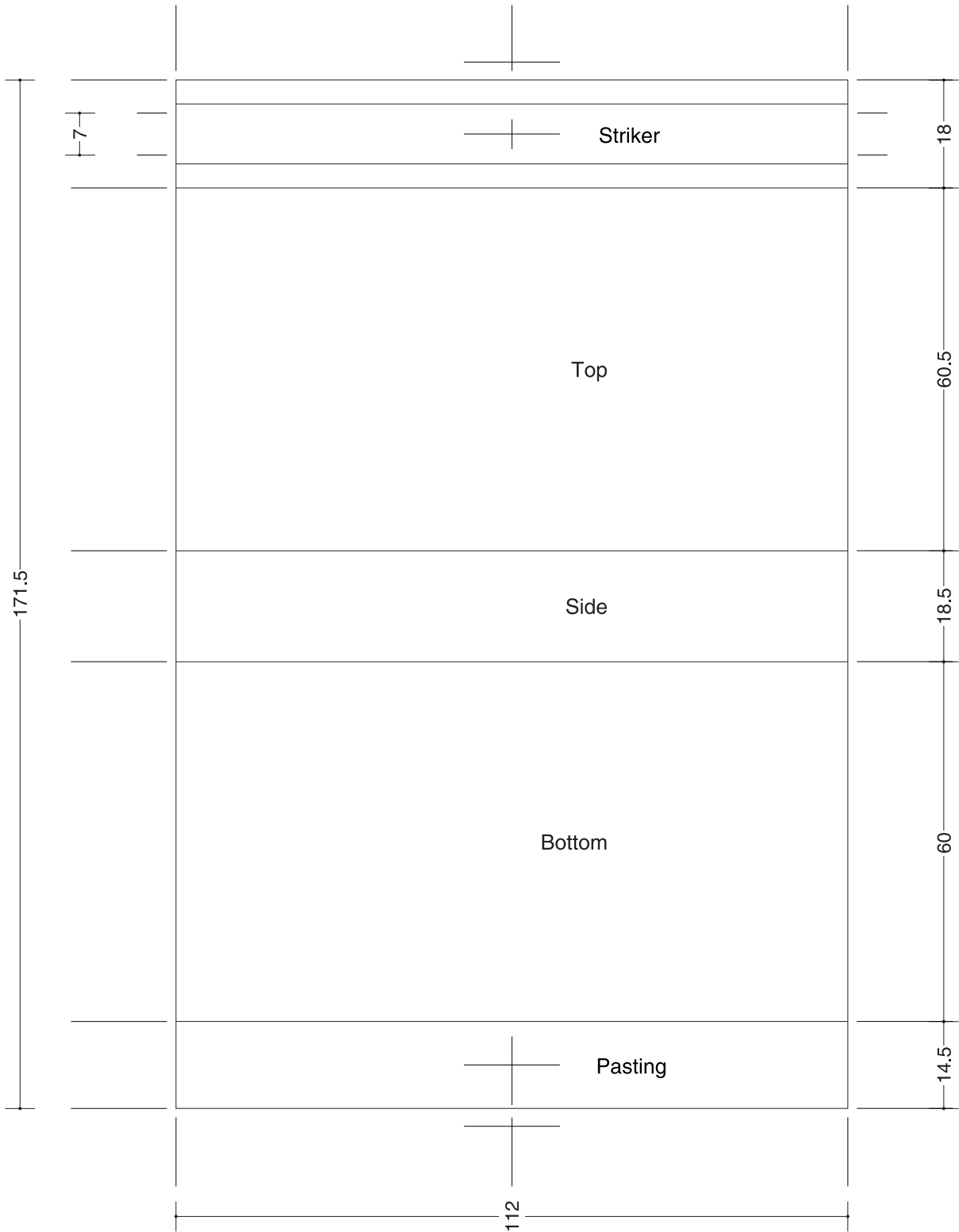
MATCHBOX DIMENSION CHART · SCALE 1/1 · UNIT m/m
