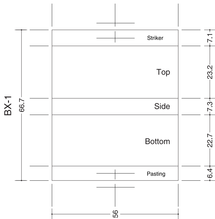
MATCHBOX DIMENSION CHART · SCALE 1/1 · UNIT m/m
