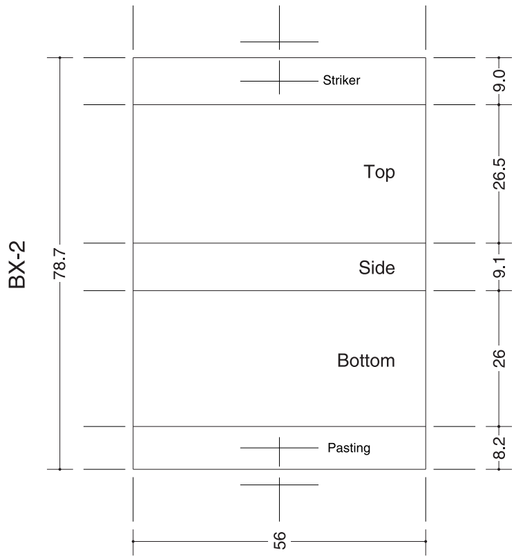
MATCHBOX DIMENSION CHART · SCALE 1/1 · UNIT m/m
