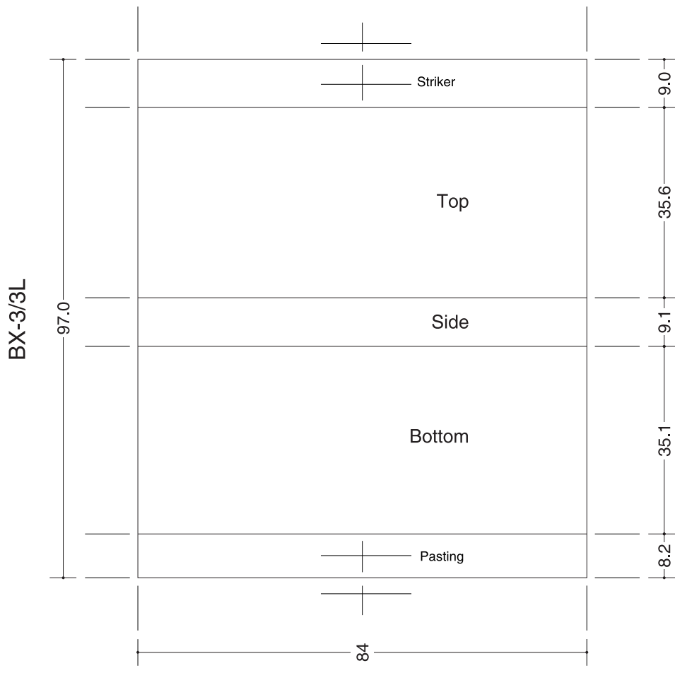
MATCHBOX DIMENSION CHART · SCALE 1/1 · UNIT m/m
