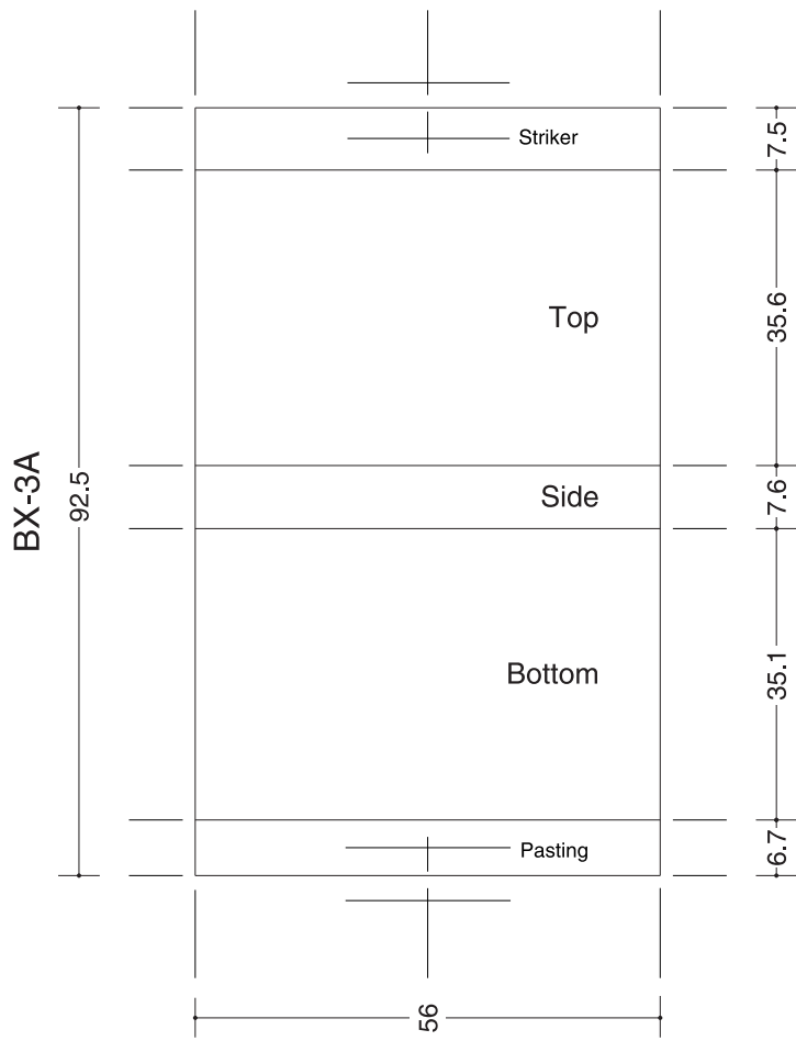
MATCHBOX DIMENSION CHART · SCALE 1/1 · UNIT m/m
