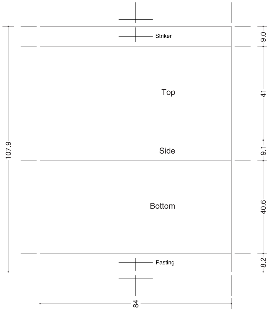
MATCHBOX DIMENSION CHART · SCALE 1/1 · UNIT m/m
