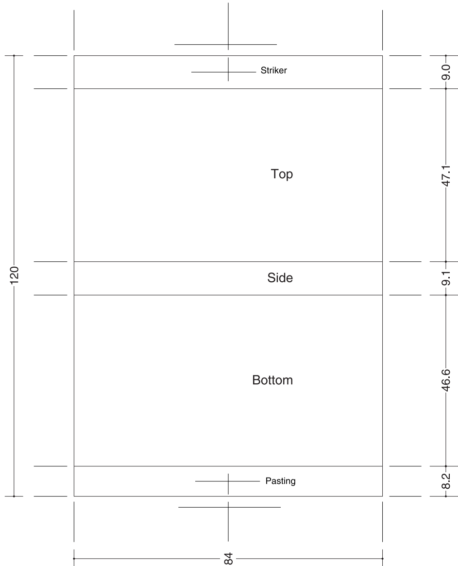
MATCHBOX DIMENSION CHART · SCALE 1/1 · UNIT m/m
