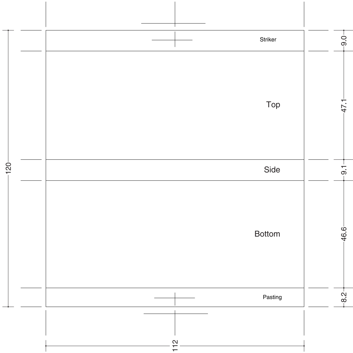
MATCHBOX DIMENSION CHART · SCALE 1/1 · UNIT mm
