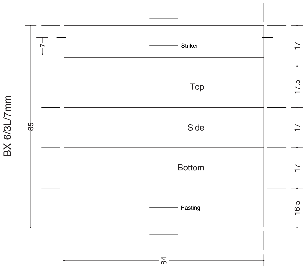
MATCHBOX DIMENSION CHART · SCALE 1/1 · UNIT m /m
