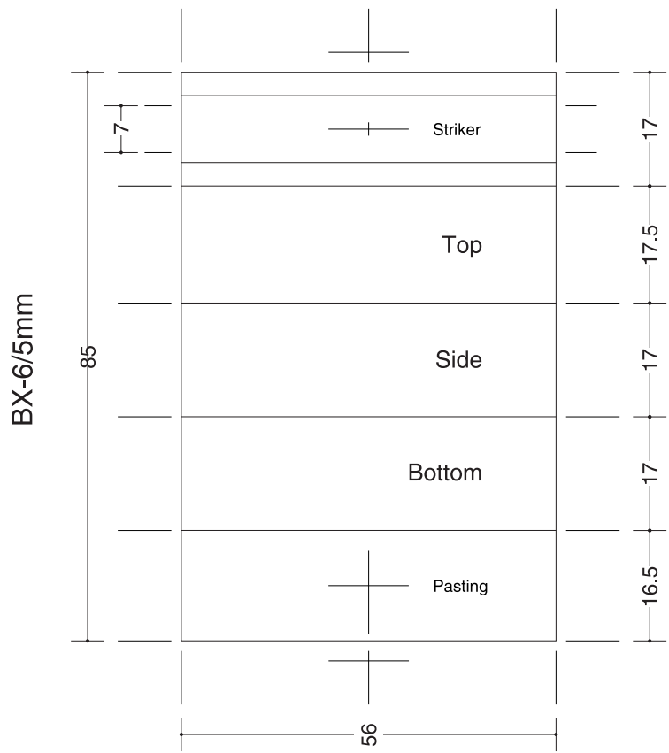
MATCHBOX DIMENSION CHART · SCALE 1/1 · UNIT m /m
