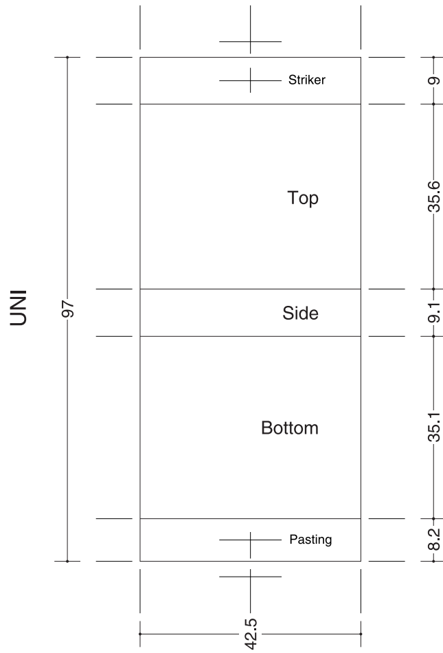
MATCHBOX DIMENSION CHART · SCALE 1/1 · UNIT m/m
